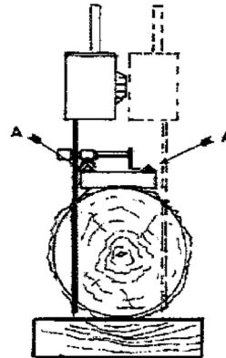
YHDISTÄ KAKSI KISKOA 2' X 6'-KOKOISEEN LANKKUUN, VALMIIN HIRREN MITTOIHIN. SAHAA SITTEN MOOTTORISAHALLASI, JOHON ON KIINNITETTY PIENI SAHALAITOS, ENSIN TOINEN PUOLI JA PALAA SAHAAMALLA TOINEN PUOLI.
