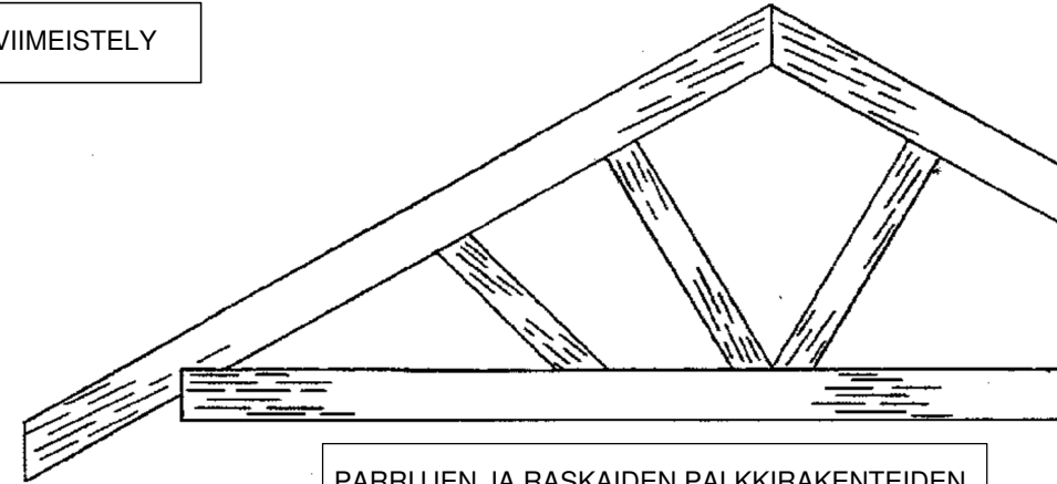
PARRUJEN JA RASKAIDEN PALKKIRAKENTEIDEN KAIKENTYYPPISEN SAHAAMINEN
