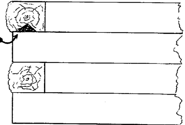
PINOTTU HIRSIRAKENNELMA
