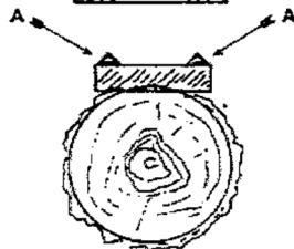
YHDISTÄ KAKSI KISKOA 2' X 6'-KOKOISEEN LANKKUUN, VALMIIN HIRREN MITTOIHIN. SAHAA SITTEN MOOTTORISAHALLASI, JOHON ON KIINNITETTY PIENI SAHALAITOS, ENSIN TOINEN PUOLI JA PALAA SAHAAMALLA TOINEN PUOLI.
